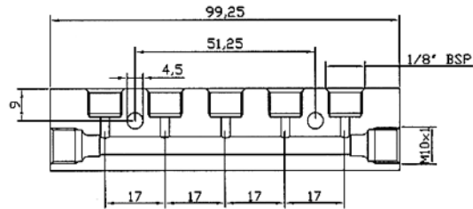
5 Auslässe Teile-Nummer: 3071305
