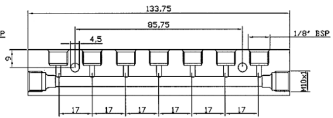
7 Auslässe Teile-Nummer: 3071307
