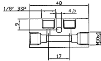
2 Auslässe Teile-Nummer: 3071302
