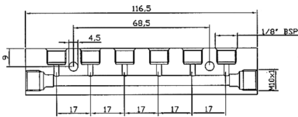
6 Auslässe Teile-Nummer: 3071306
