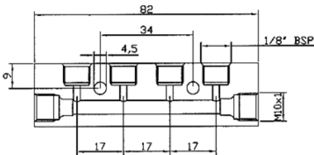
4 Auslässe Teile-Nummer: 3071304
