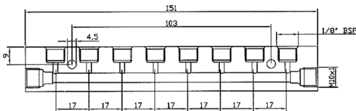
8 Auslässe Teile-Nummer: 3071308
