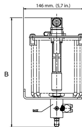
Бак 3 литра
