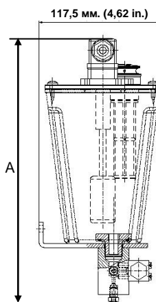
Бак 1 литр
